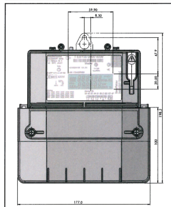
Drehstromzähler Q3AXXXX4, Q3AXXXX5 mit Klemmendeckel „60“
