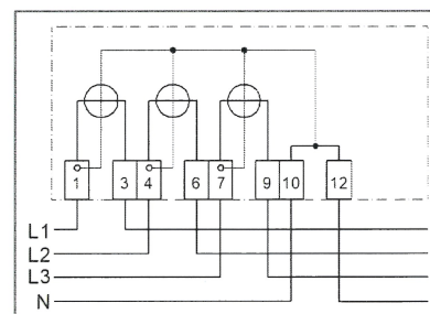
Abb. oben: Anschlusschaltbild 4000 ohne Tarifschaltung, ohne Zusatzklemmen.
