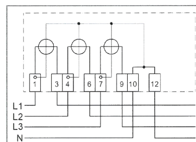
Abb. oben: Anschlusschaltbild 4100 ohne zusätzliche Klemmen, Tarifschaltung nur über die MSB-Schnittstelle.
