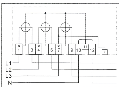
Abb. oben: Anschlusschaltbild 4000 mit zusätzlichen Klemmen 7', 11 (gilt für: Q3AX10X0)
