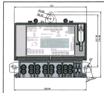
Drehstromzähler Q3AXXXX4, Q3AXXXX5 ohne Klemmendeckel
